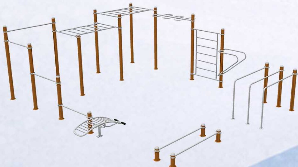
NT 157G Área: 12,5 x 12,5 m Usuarios: 13
