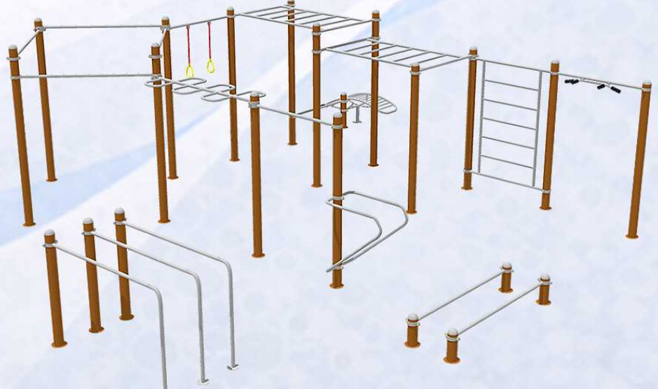
NT 177G Área: 12,8 x 10,8 m Usuarios: 17
